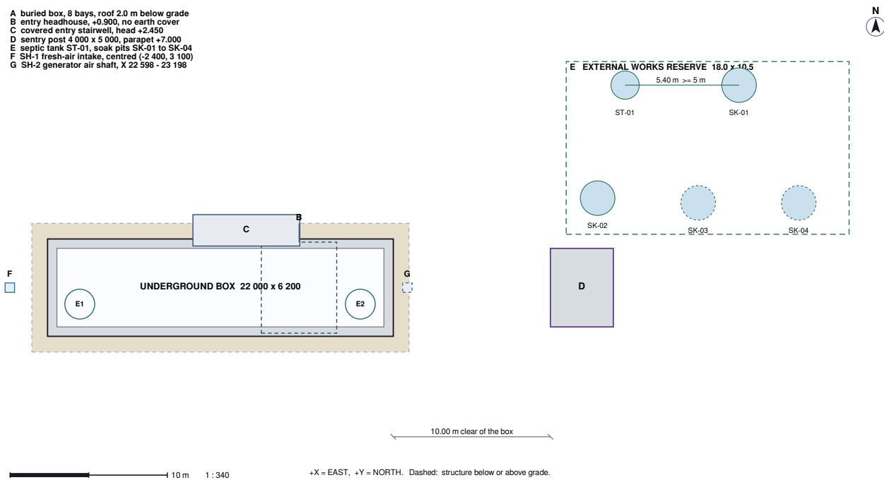
Fig 2.1 : Site Layout Plan
